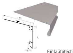
Einlaufblech
