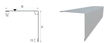
Außenecke
