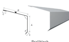
Prallblech
